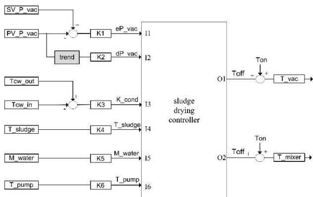
Slika 4: Shema regulatorja za sušenje mulja.
